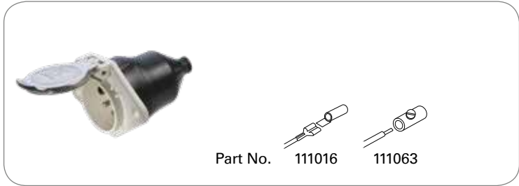
7P/24V Socket (ISO 3731 - Type S)
