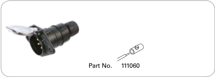
7P/24V Plug (ISO 1185 - Type N)
