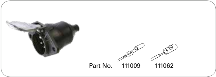
7P/24V Socket (ISO 1185 - Type N)
