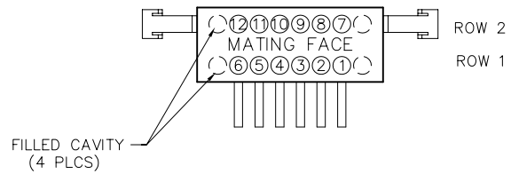
RECEPTACLE MA-2C1-012-435-A5300
