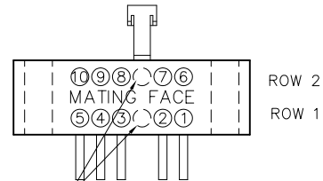
RECEPTACLE MA-2E1-010-435-ALC00
